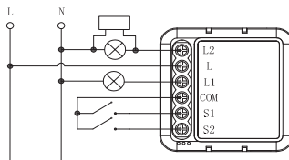
Układ schodowy
