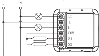
Podłączenie urządzenia
