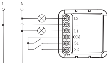
Podjedynczy przełącznik
