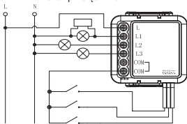
Układ schodowy
