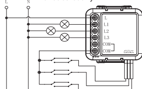
Układ schodowy
